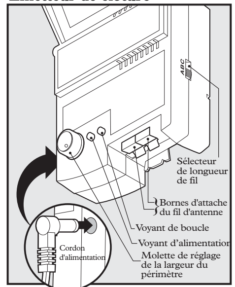
Émetteur de clôture
